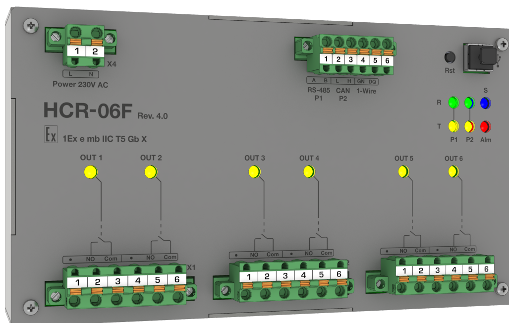
Рисунок 1.1 – Внешний вид устройства HCR-06F Ex
