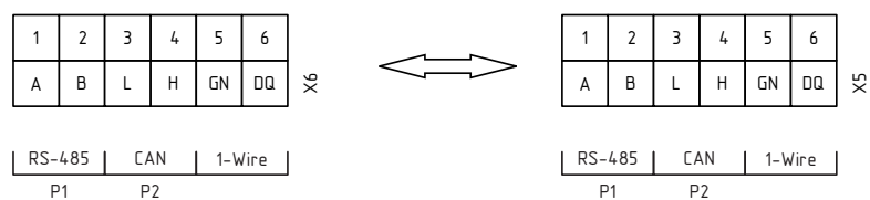
Рисунок Ж.5 – Интерфесы связи
