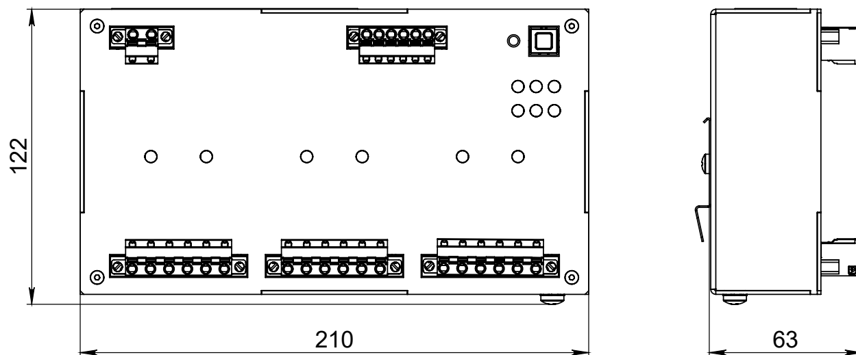
Рисунок Б.1 – Габаритные размеры HCR-06F Ex Rev.3.0, Rev.4.0
