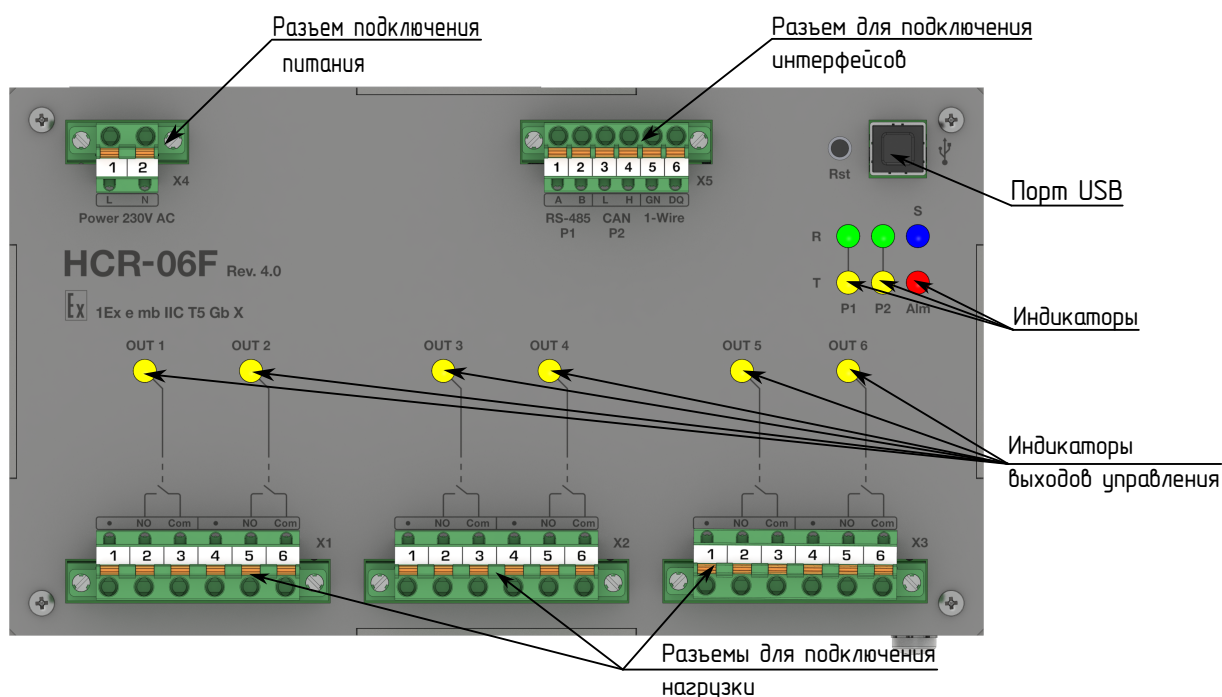
Рисунок 1.2 – Назначение основных элементов на лицевой панели
