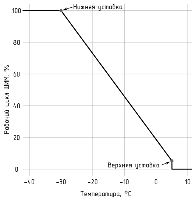
Рисунок 1.4 – Режим работы «Пропорциональный ШИМ»
