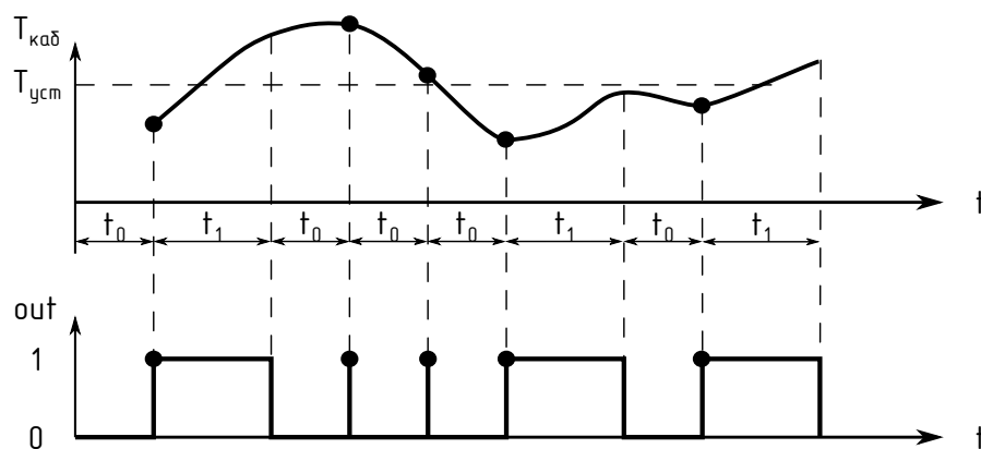
Рисунок 1.5 – Режим работы «По току саморегулирующегося кабеля»
