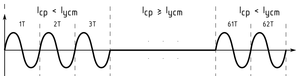
Рисунок 1.7 – Режим «Ограничение тока»
