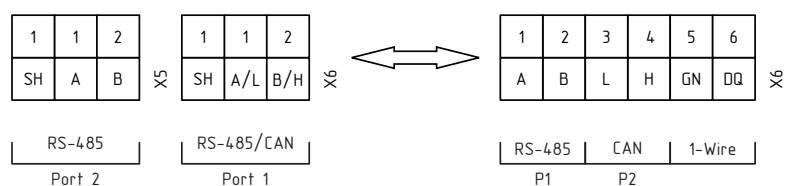
Рисунок Ж.4 – Интерфесы связи
